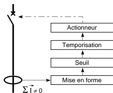
Fig. 24 : schéma fonctionnel d'un DDR.
