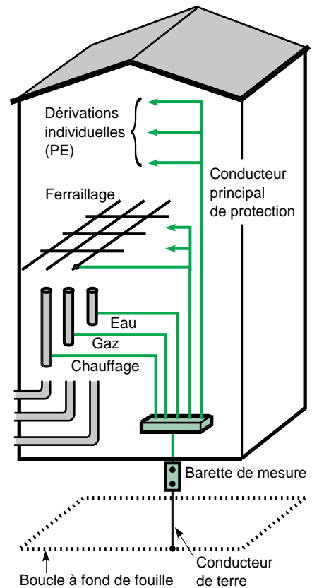
Fig. 4 : équipotentialité dans un immeuble.
