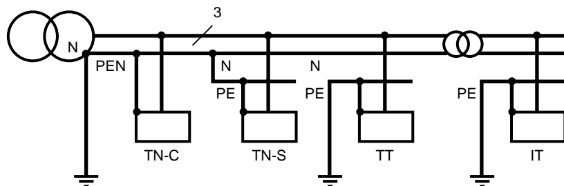
Fig. 6 : exemple de coexistence entre les divers SLT.
